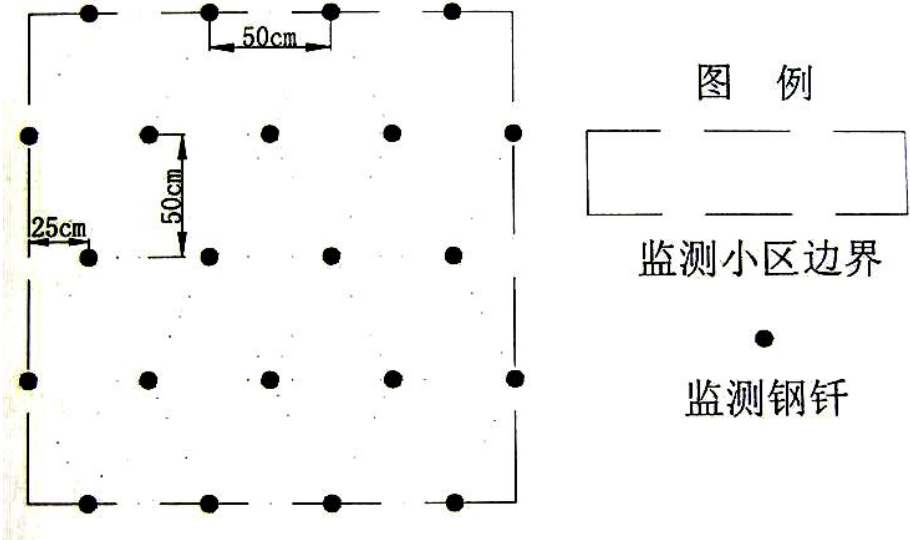
图 2.1-3 测钎法示意图
