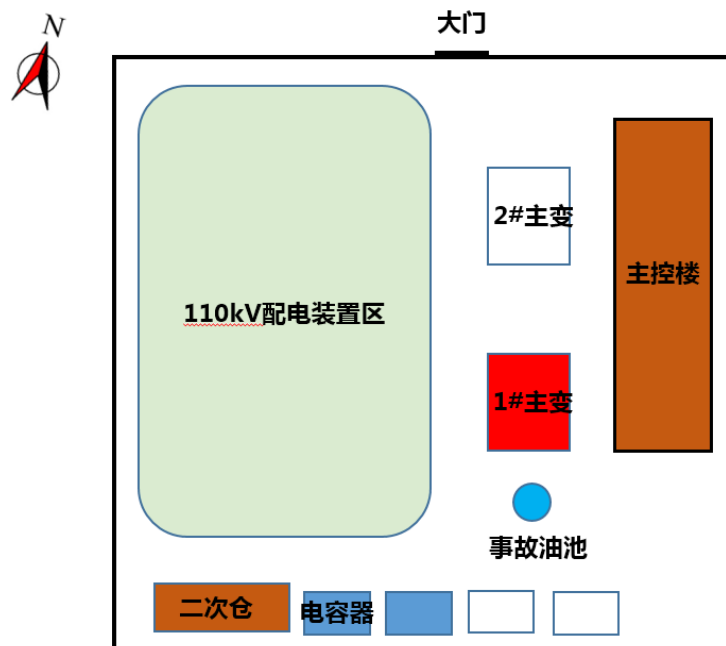
图 2 山门 110kV 变电站总平面布置示意
