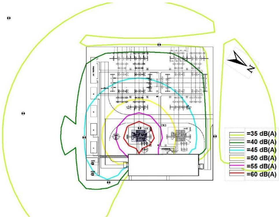
图 10 山门 110kV 变电站本期规模噪声预测等值线图
